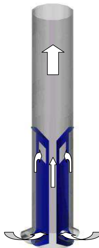
2. ábra - légáramok útja a szellőzőcsatornában
