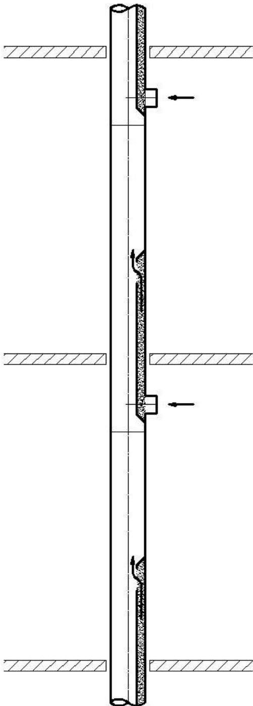
3. ábra – rendszer-összeállítás szintenkénti egy csatlakozással
