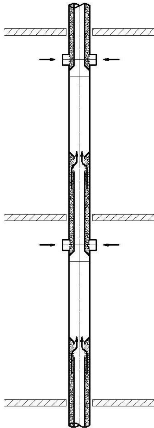
4. ábra – rendszer-összeállítás szintenkénti két csatlakozással
