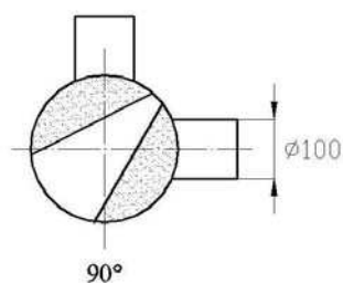
1. ábra - keresztmetszet dupla csatlakozással, 90°-os csonkelhelyezéssel
