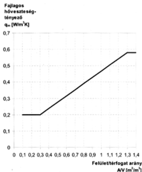
1. ábra: A fajlagos hővesztés-tényező követelményértéke
